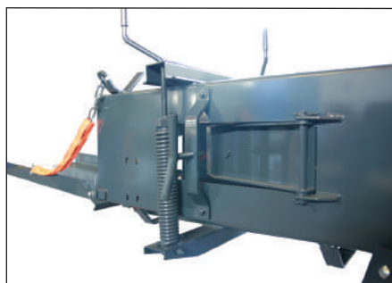
Système de compression à quatre directions pour obtenir des balles plus uniformes
